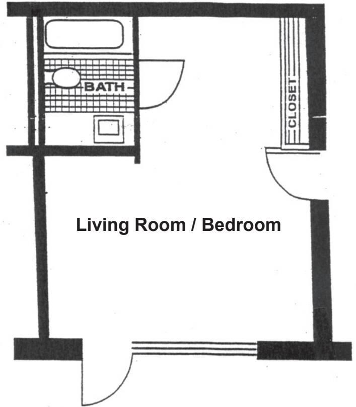
The Rose-Marie (336 s.f.)
